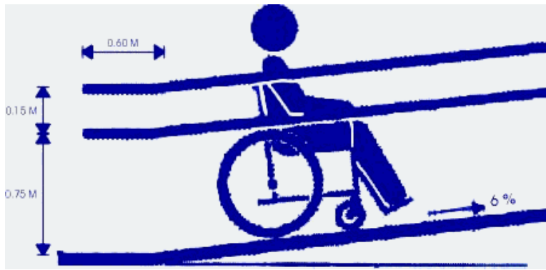
RAMPAS DE ACCESOS A BANQUETAS Y EDIFICACIONES.
